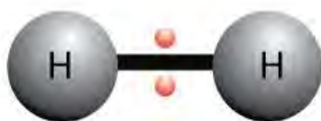
H_2 molecule
