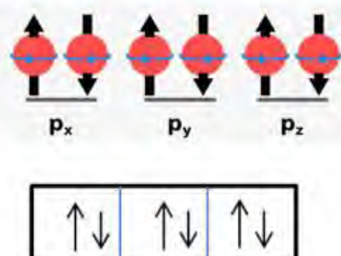
Fig: diamagnetic
