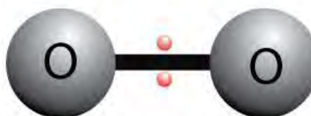
O_2 molecule
